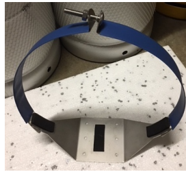
Artikel nr 153 Hållare för tankflaska 11kg o 14kg Rostfritt utförande med vajer för fastsättning av tankflaskan
